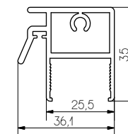
PROFILO INFISSO ORIZZONTALE
