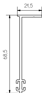
PROFILO INTERNO GUIDA
