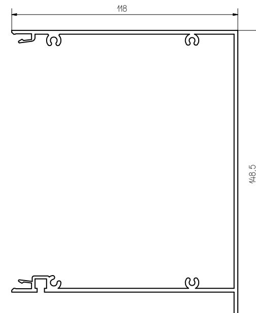
PROFILO CASSONETTO
