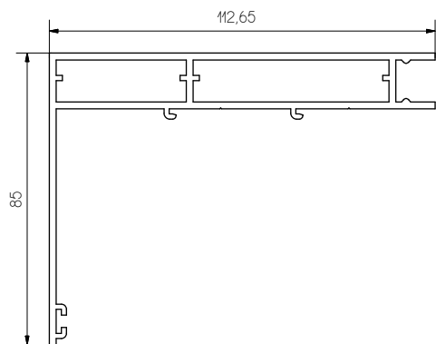
PROFILO GUIDA
