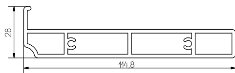
PROFILO DI BASE
